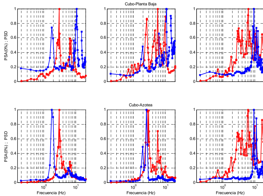
Figura 11: Espectros de potencia experimentales y PSA (0%) teóricos correspondientes al cubo de elevator-escaleras. Renglón 1: planta baja, y renglón 2: azotea. De izquierda a derecha: movimientos en la dirección longitudinal, transversal y vertical en las columnas 1, 2, y 3, respectivamente. Azul: experimental. Rojo: teórico.
